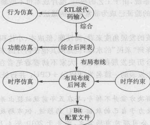
图 1.2 FPGA/CPLD 网表生成
