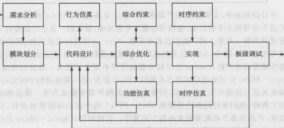
图 1.1 FPGA/CPLD 开发流程
