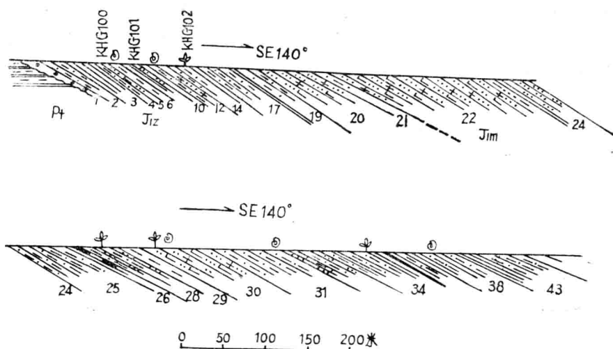
插图7 文家市剖面示意图
