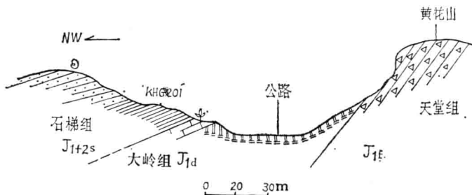
插图4 广西钟山西湾平桂矿务局公路剖面示意图
