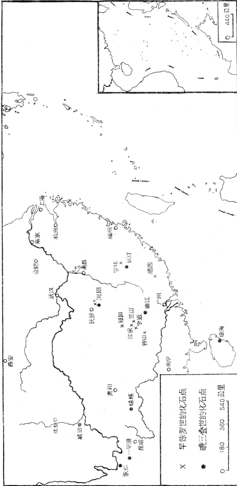
插图 1 华南昆虫化石产地分布简图
