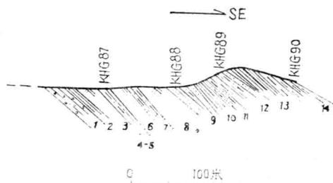
插图 5 造上村造上组剖面示意图(仿煤炭部地勘所)*
