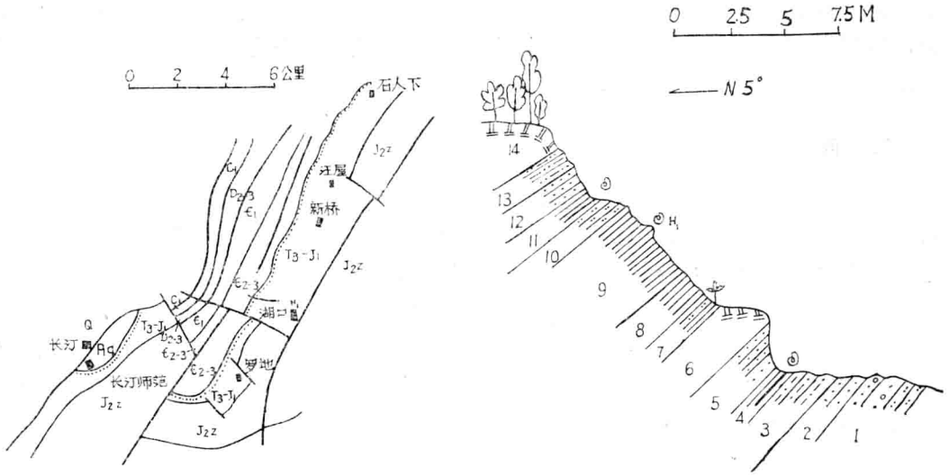
插图 2, 3 福建长汀湖口昆虫化石(H 1 )点位置和剖面示意图
