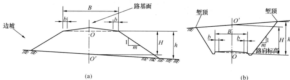
图 1-2 路基本体
