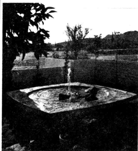
圖A：此一造型突出的噴泉是利用易於彎曲的銅管焊接上普通的噴嘴，來造成特殊的效果。突出水面而彎曲的銅管及細長的水柱在空中龍飛鳳舞，頗有立體雕塑的風格。盛水的鐵盤已經防銹處理過，但仍須適時清理滋生的藻類。
