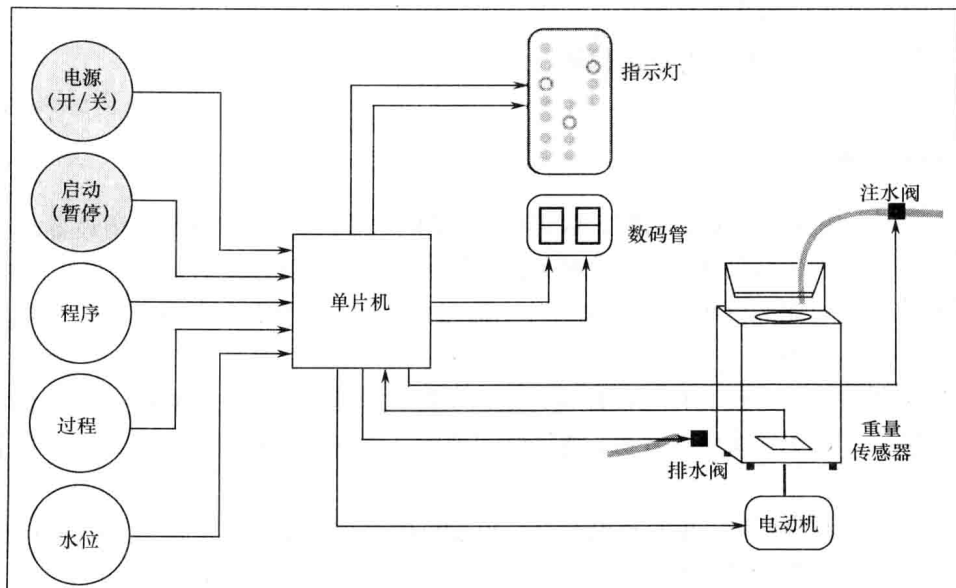
图 1.1 洗衣机的单片机控制图
