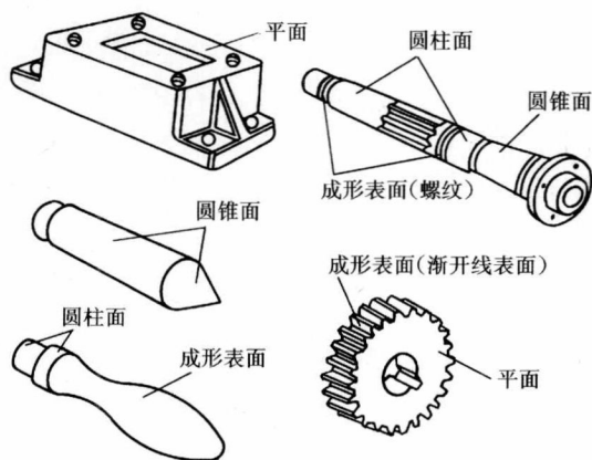
图 1-1 机器零件上常用的各种典型表面
