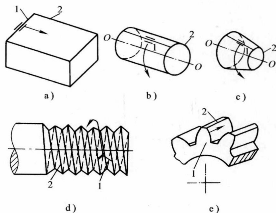
图 1-2 零件表面的形成
