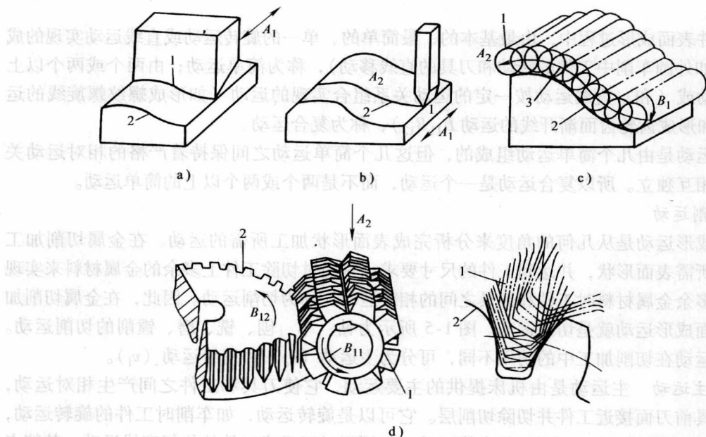
图 1-3 形成发生线的四种方法及运动
