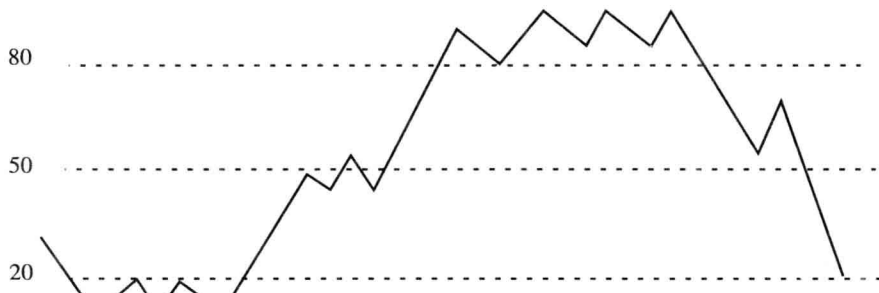
图 1-1 RSI (KDJ) 超买超卖示意图
