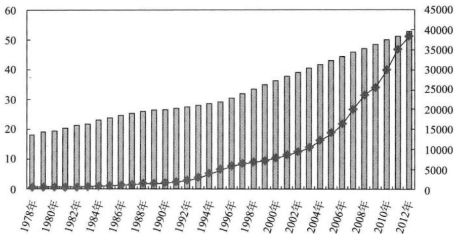
图 1 中国 1978—2012 年城镇化率与人均 GDP 的曲线变化图
