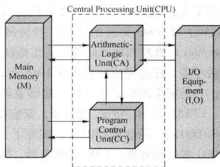
图 1-4 冯·诺伊曼体系结构
