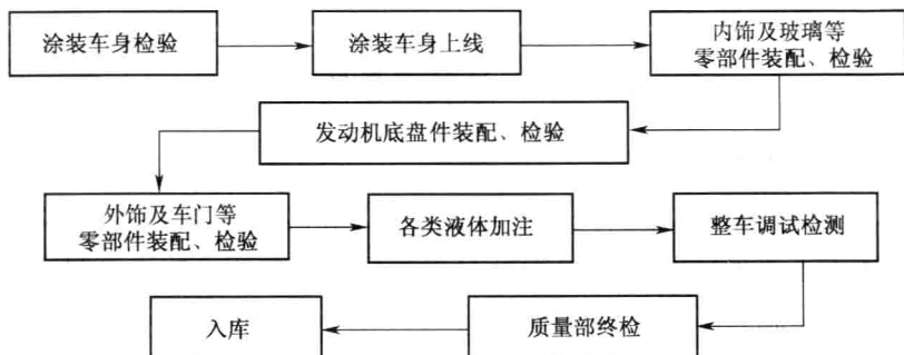
图 1-1 总装工艺流程
