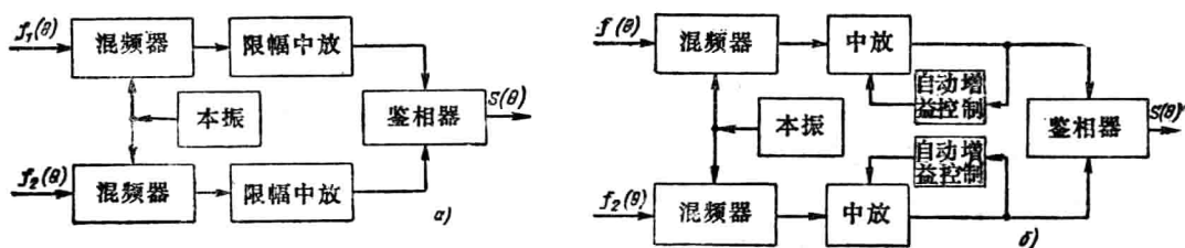
图1-5 相位角度鉴别器的方框图
