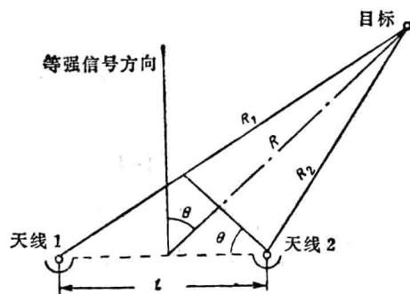
图1-2 相位定向法单脉冲雷达中角座标的测定
