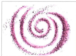
涡状星云
