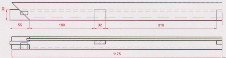
06 大边
