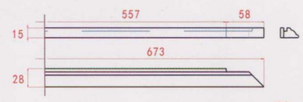
08 侧压线
