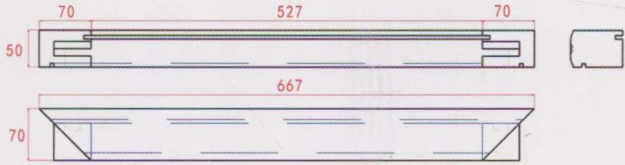
02 抹头
