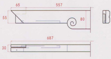
07 侧牙板
