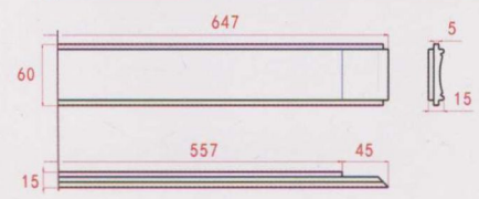
09 侧束腰
