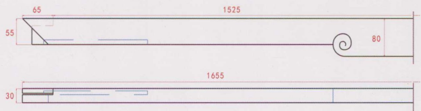
07 牙板
