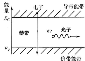
图 1.1.4 能带图
