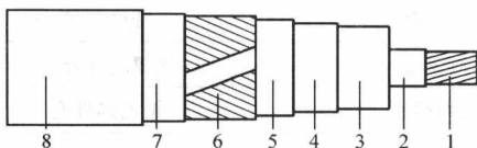
图 1-5 单芯交联聚乙烯绝缘电缆
