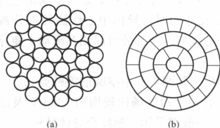
图 1-7 圆形导体紧压前后的截面图 (a) 导体线芯紧压前；(b) 导体线芯紧压后
