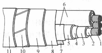
图 1-4 三芯分相铅套油纸绝缘铠装电缆
