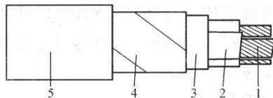
图 1-2 三芯聚氯乙烯绝缘内钢带铠装电缆
