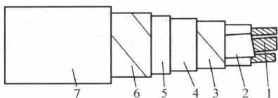
图 1-1 1kV 三芯油浸纸绝缘电缆
