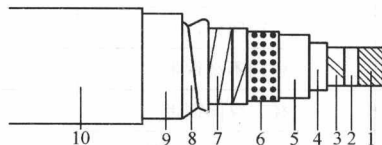
图 1-6 单芯纸绝缘皱纹铝套充油电缆
