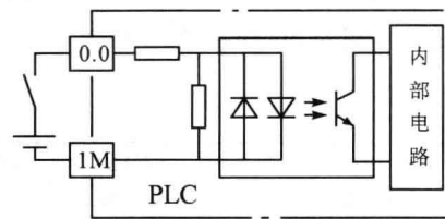
图 1-3 输入电路
