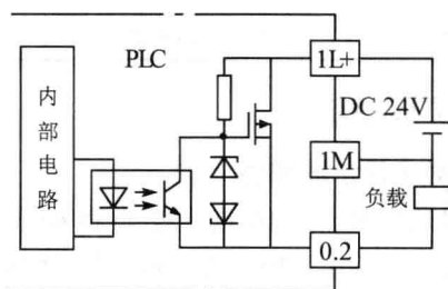
图 1-5 场效应晶体管输出电路
