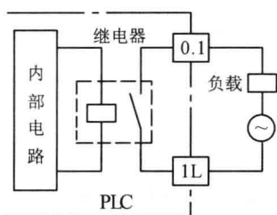
图 1-4 继电器输出电路
