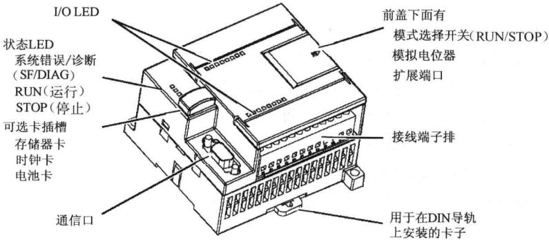
图 1-2 S7-200 CPU 模块的外形图
