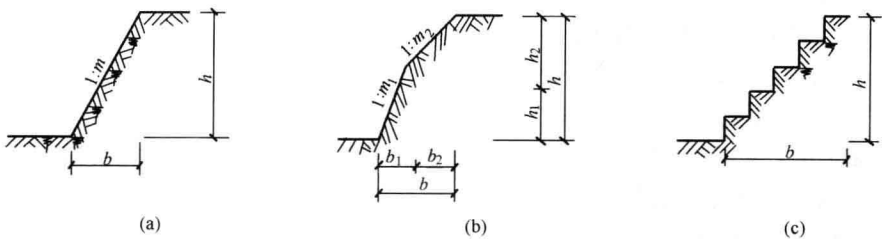
图 1-1 土方放坡形式 (a) 直线形；(b) 折线形；(c) 阶梯形
