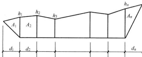
图 1-10 断面法
