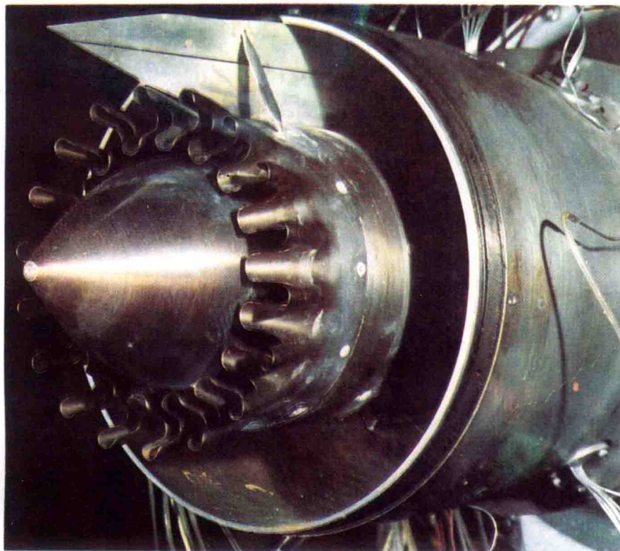
GE公司高效节能 发动机排气混合器
