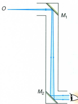
圖 1.2k 潛望鏡示意圖
