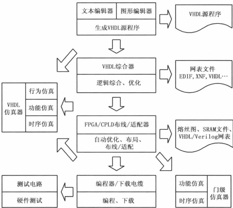
图 1-1 EDA 工程设计流程图
