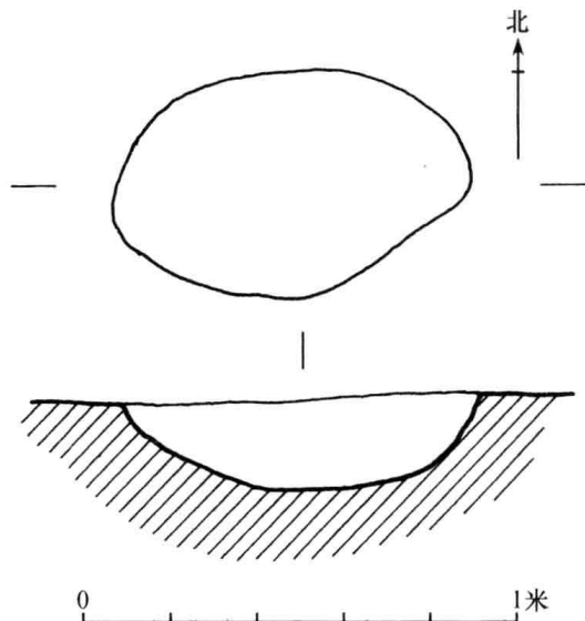
图五 2012XQZH3平、剖面图
