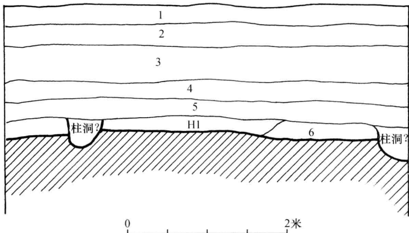
图九 2012XQST1西壁剖面图
