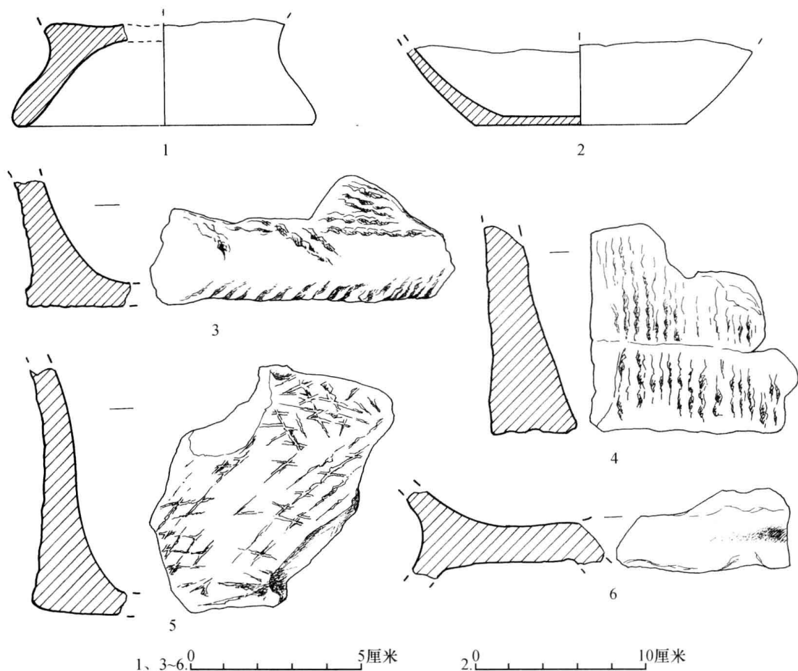
图七 赵家河坝遗址出土陶器
