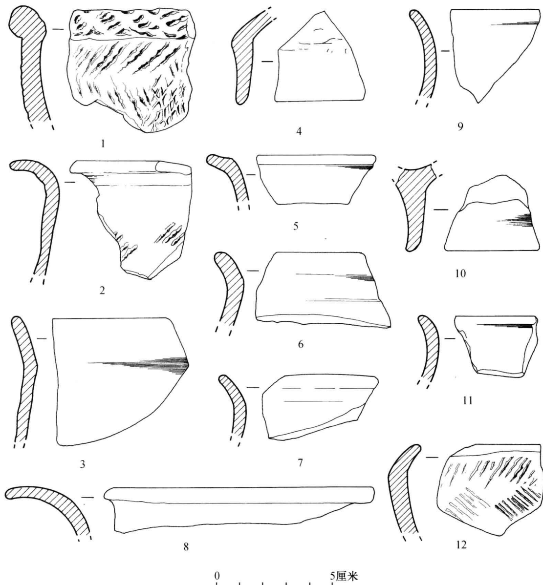
图六 赵家河坝遗址出土陶器
