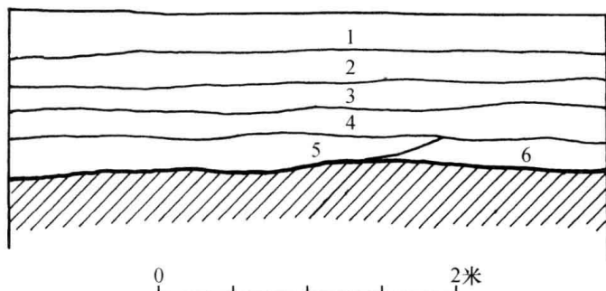
图三 2012XQZT1北壁剖面图
