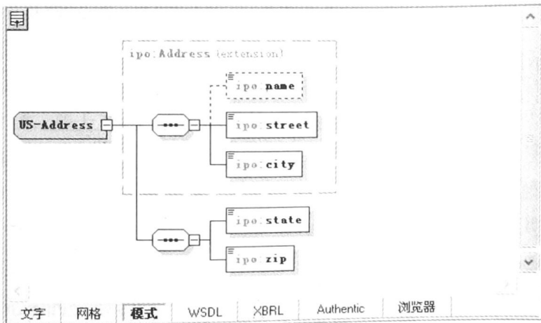
图 1-5 以模式视图显示 Schema 文档
