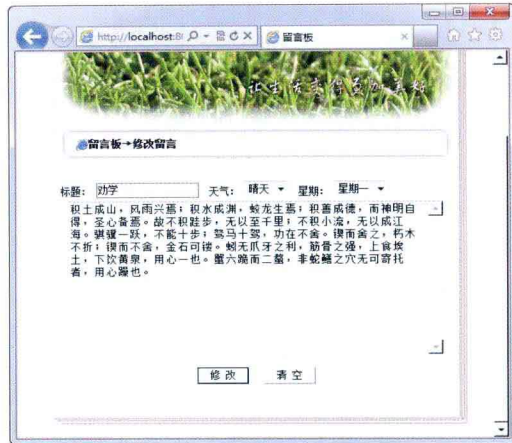
修改留言
