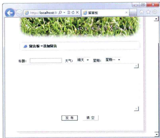
添加留言
