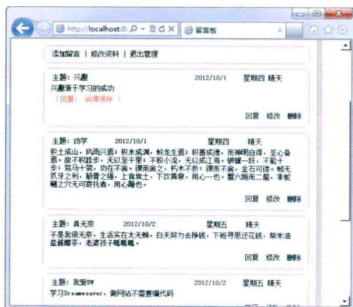
留言管理
