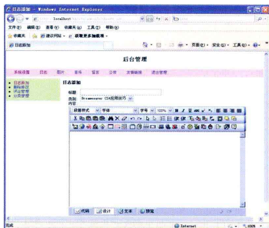
后台管理
