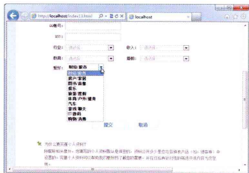
(13.4.12 节) 插入菜单
