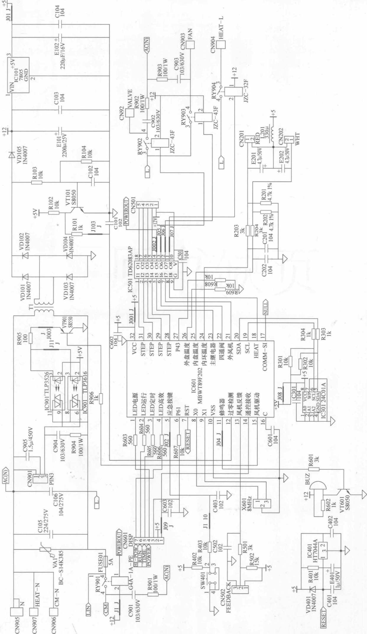
图 14-1 海信 KFR-25GW/57D、KFR-32GW/57D 型空调器的电脑板电路
