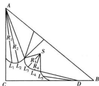
图 1.3 三元水盐系相图
