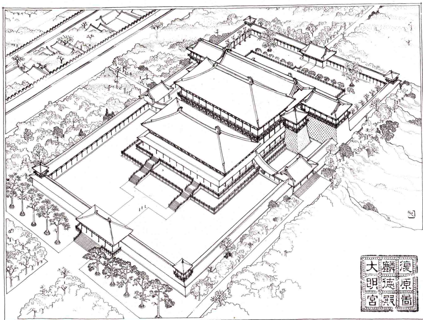
圖五 大明宮麟德殿復原圖
