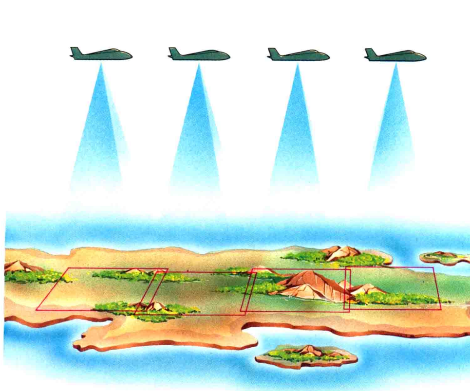
航空照相在測量及製圖上已成為一項重要的技術。上：測量飛機對地面拍攝一系列有部分重疊的照片，這些照片可再加以組合成一張照片圖。照片圖上如山頂等已知的參考點，可以用來與由傳統測量方法獲得的資料核對。
