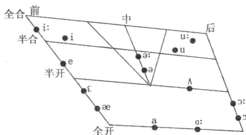
单元音发音部位示意图
