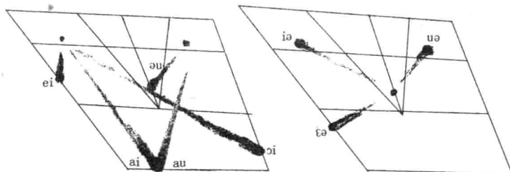
双元音滑动方向示意图
