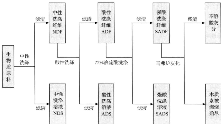
图 1-2 范氏组分分析法
