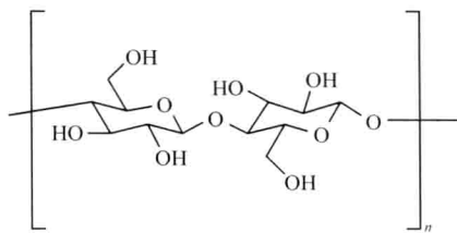
图 1-3 纤维素基本单元结构
