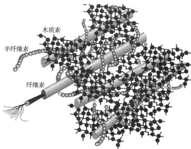
图 1-1 生物质的组成结构
