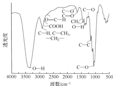
(d) 微晶纤维素红外压片谱图
