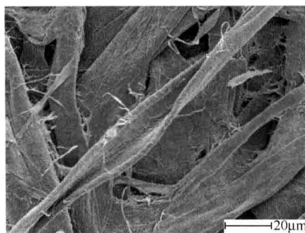
(a) 定性滤纸扫描电镜照片
