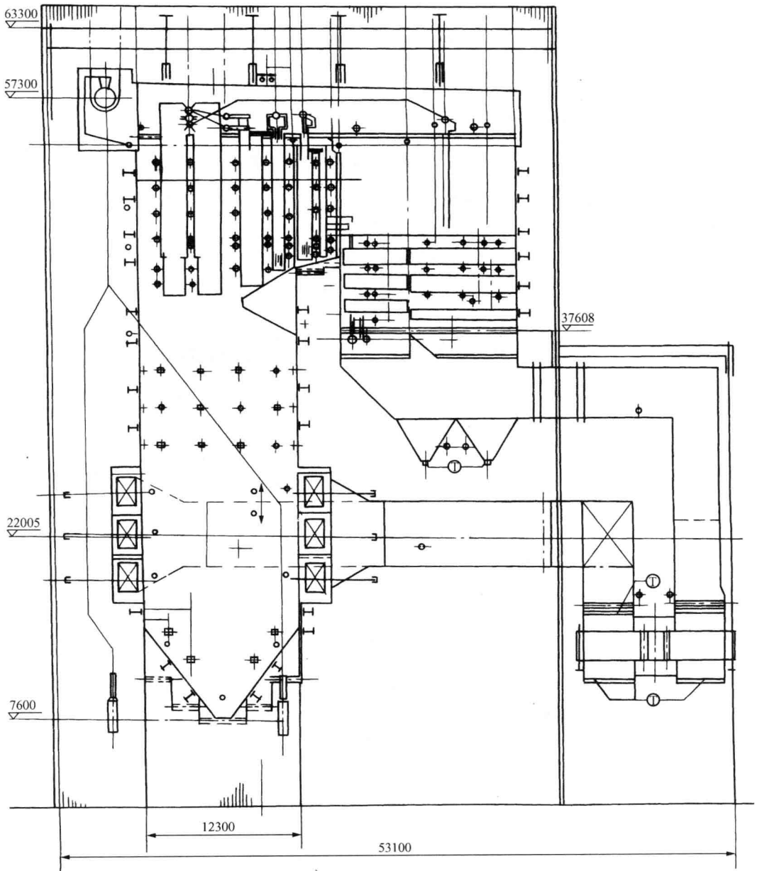
图 1-4 采用对冲燃烧方式的 300MW 自然循环锅炉
