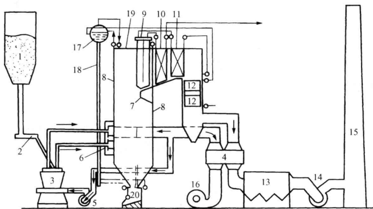
图 1-1 燃煤锅炉机组的工作过程示意
