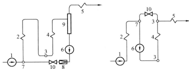
图 1-3 低倍率复合循环锅炉系统
