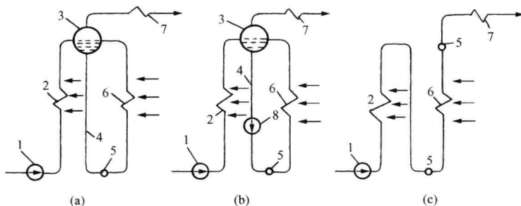
图 1-2 蒸汽锅炉蒸发部分的几种类型
