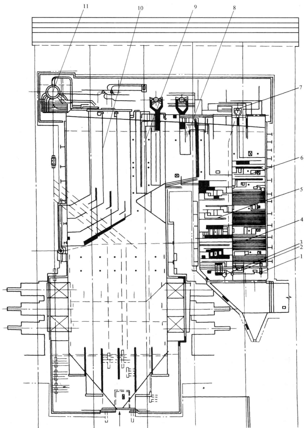
图 1-6 FW 亚临界参数 600MW 自然循环锅炉
