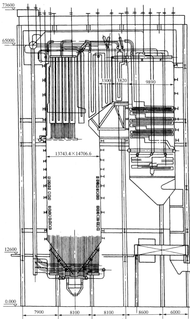
图 1-5 采用四角燃烧方式的 300MW 自然循环锅炉
