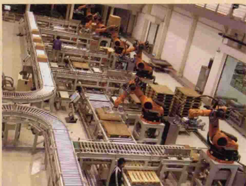
昆船设备集团码垛机器人 供稿：省经济委员会
