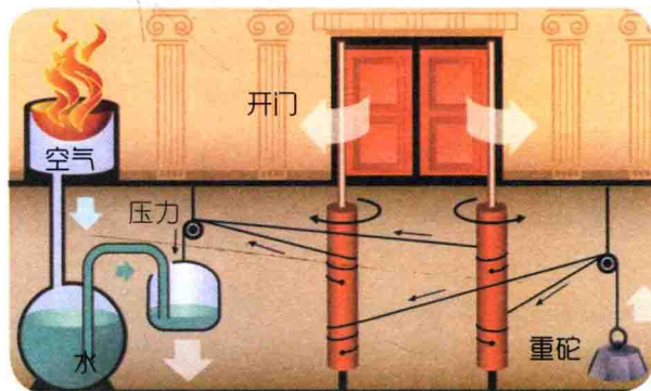
神奇自动门的机械原理图
