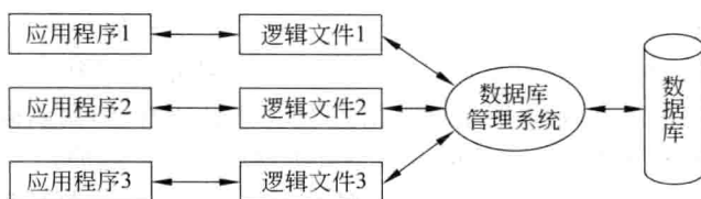
图 1-1 在数据库系统中数据与应用程序之间的关系
