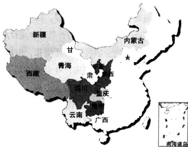
图 1-1 西部地区 12 省
