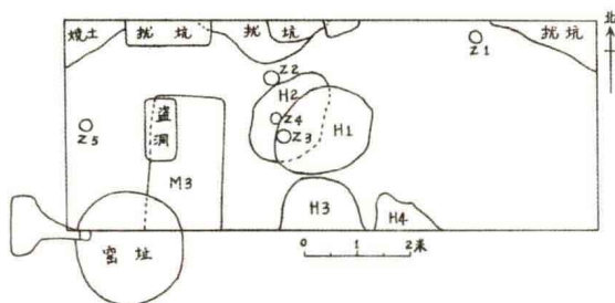
图2 探方一(T 1 )平面图
