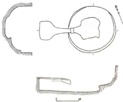
图6 窑址平、剖面图
