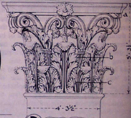
(D) PORTICO CAPITAL
