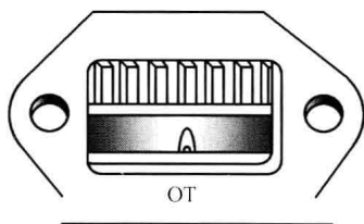
图 1-18 1 (6) 缸上止点标记
