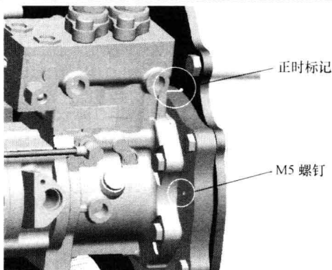
图 1-19 油泵的安装
