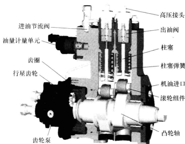
图 1-5 双柱塞高压泵结构
