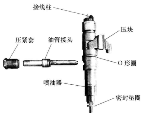
图 1-17 喷油器拆装
