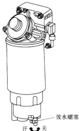
图 1-14 油水分离器上的放水螺塞
