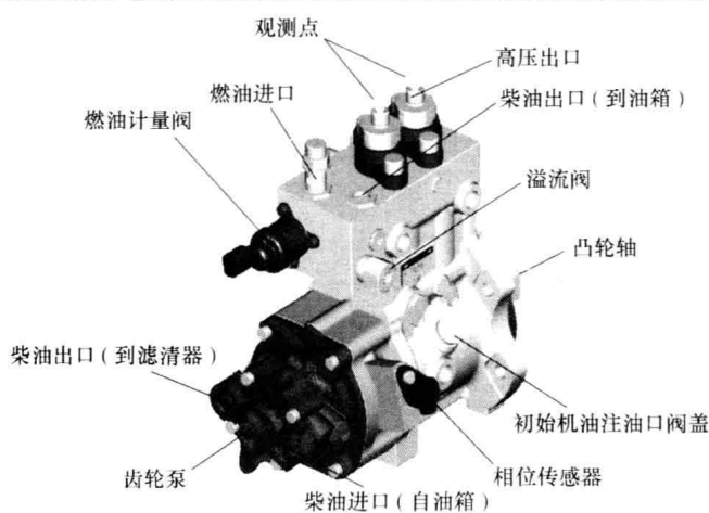
图 1-16 高压油泵性能检查
