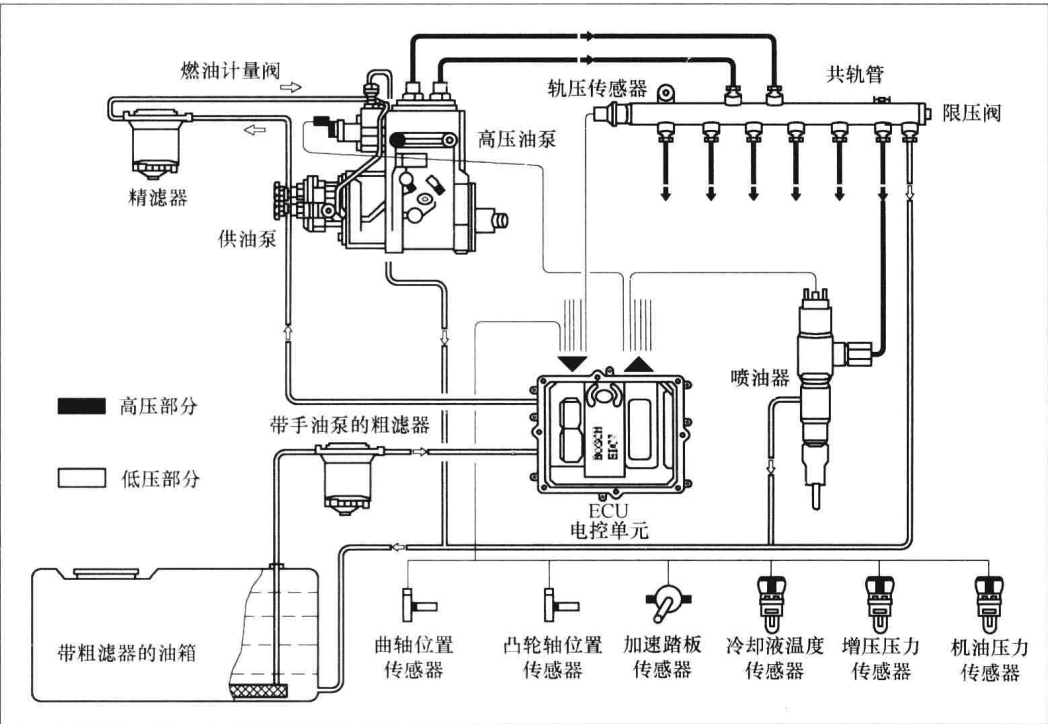
图 1-1 潍柴 WP10/12 发动机燃油回路
