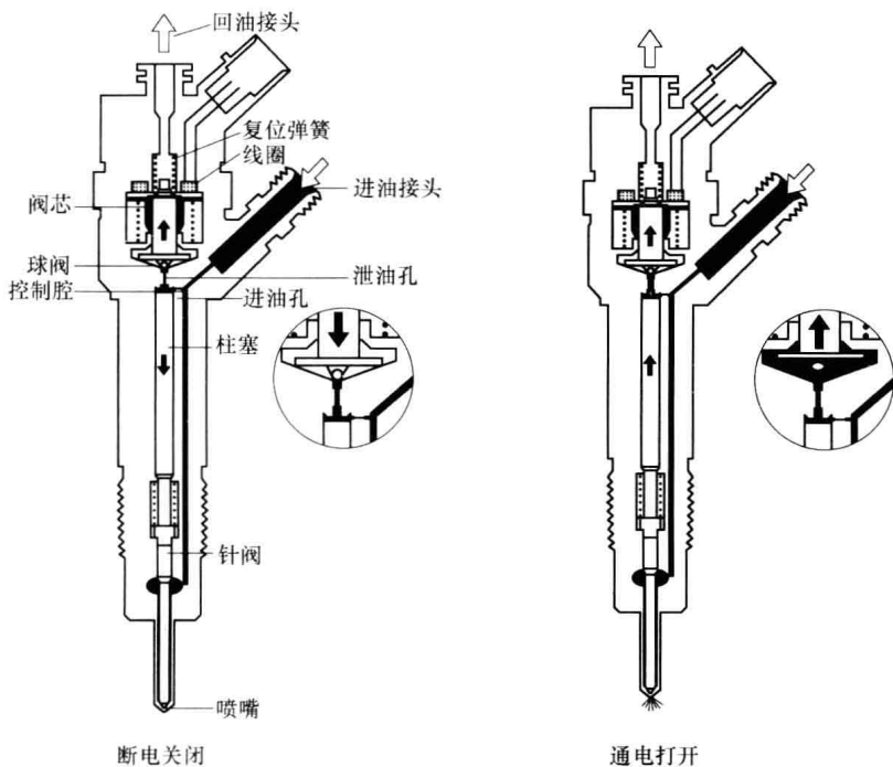
图 1-11 喷油器
