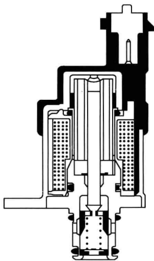
图 1-7 油量计量单元通电关闭
