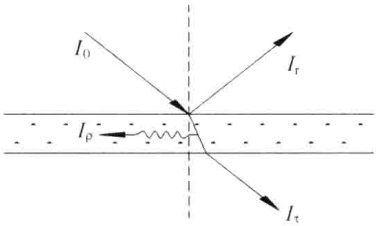
图 1-2 物体对辐射热的吸收、反射和透射示意
