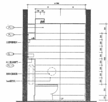
B 立面圖
