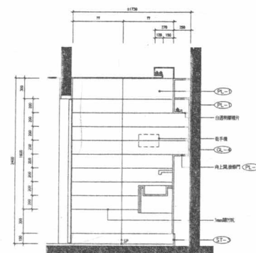
A 立面圖
