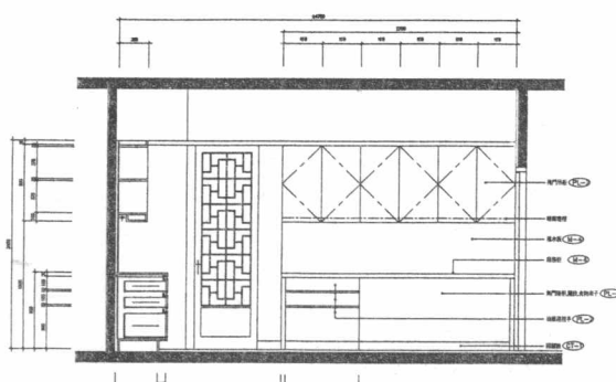
D 餐廳立面圖
