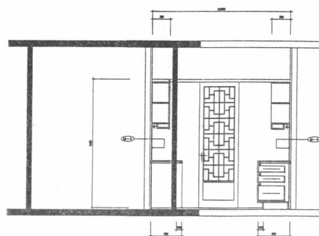
A 餐廳立面圖
