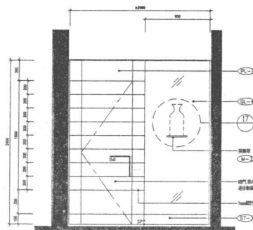
A 立面圖
