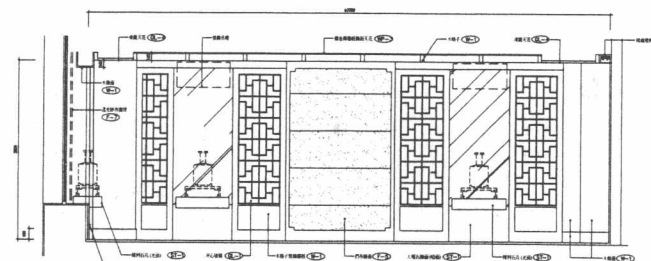
1 貴賓房立面圖
