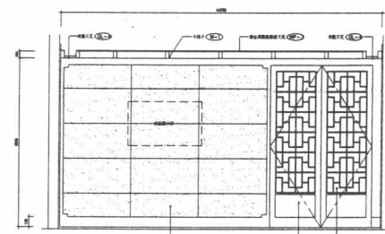
6 貴賓房立面圖
