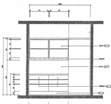
C 餐廳立面圖
