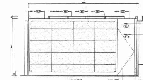
7 貴賓房立面圖
