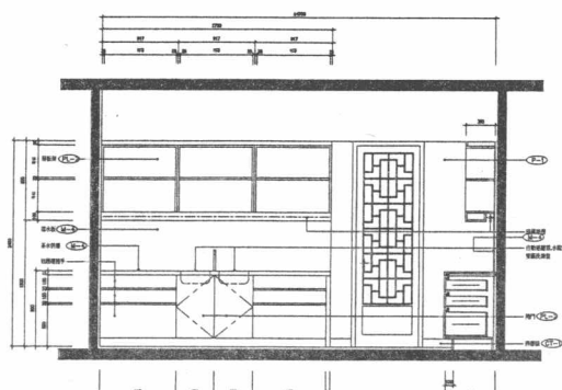
B 餐廳立面圖
