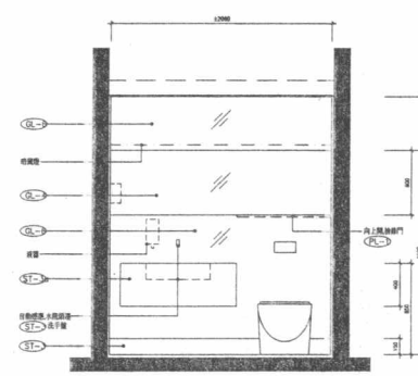
B 立面圖
