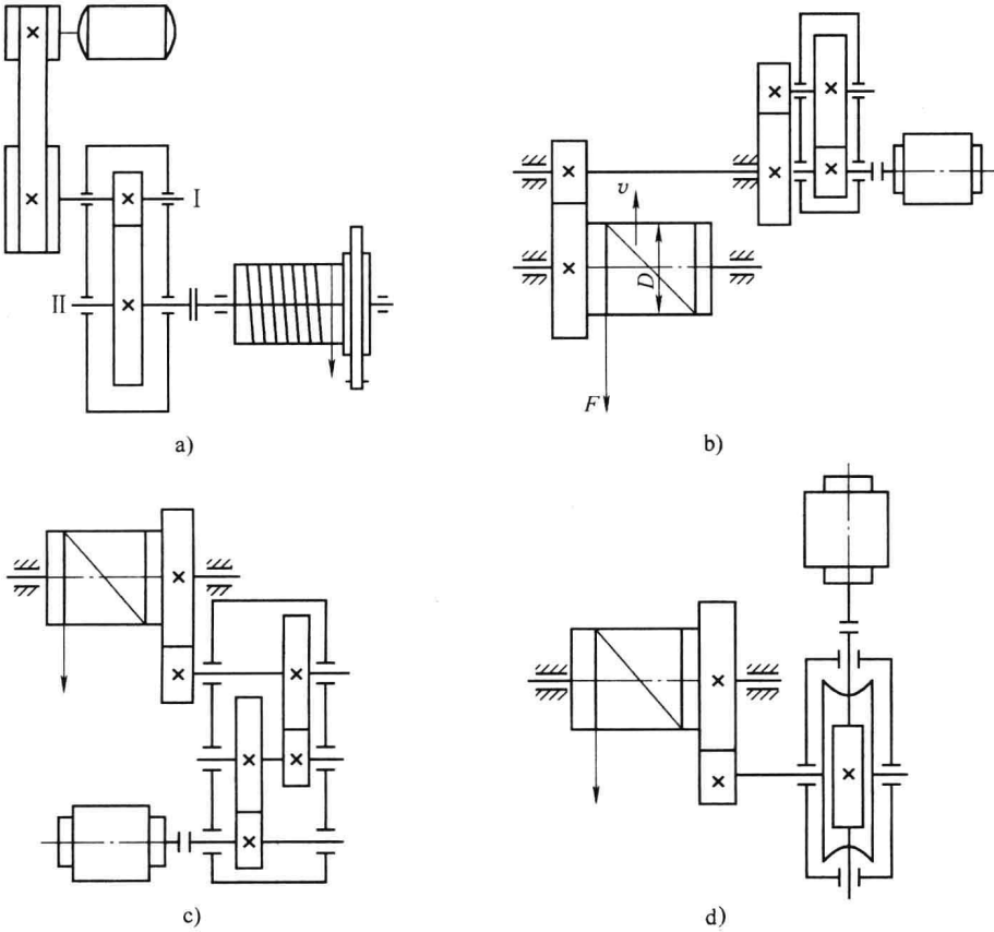
图 1-6 卷扬机传动方案
