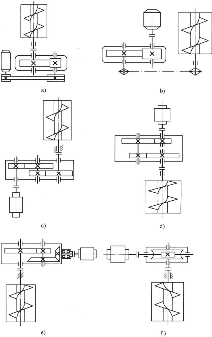
图 1-4 螺旋输送机传动方案
