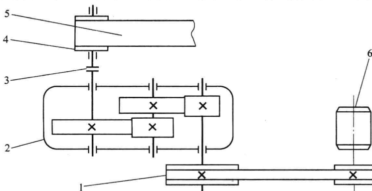
图 1-1 带式输送机传动装置
