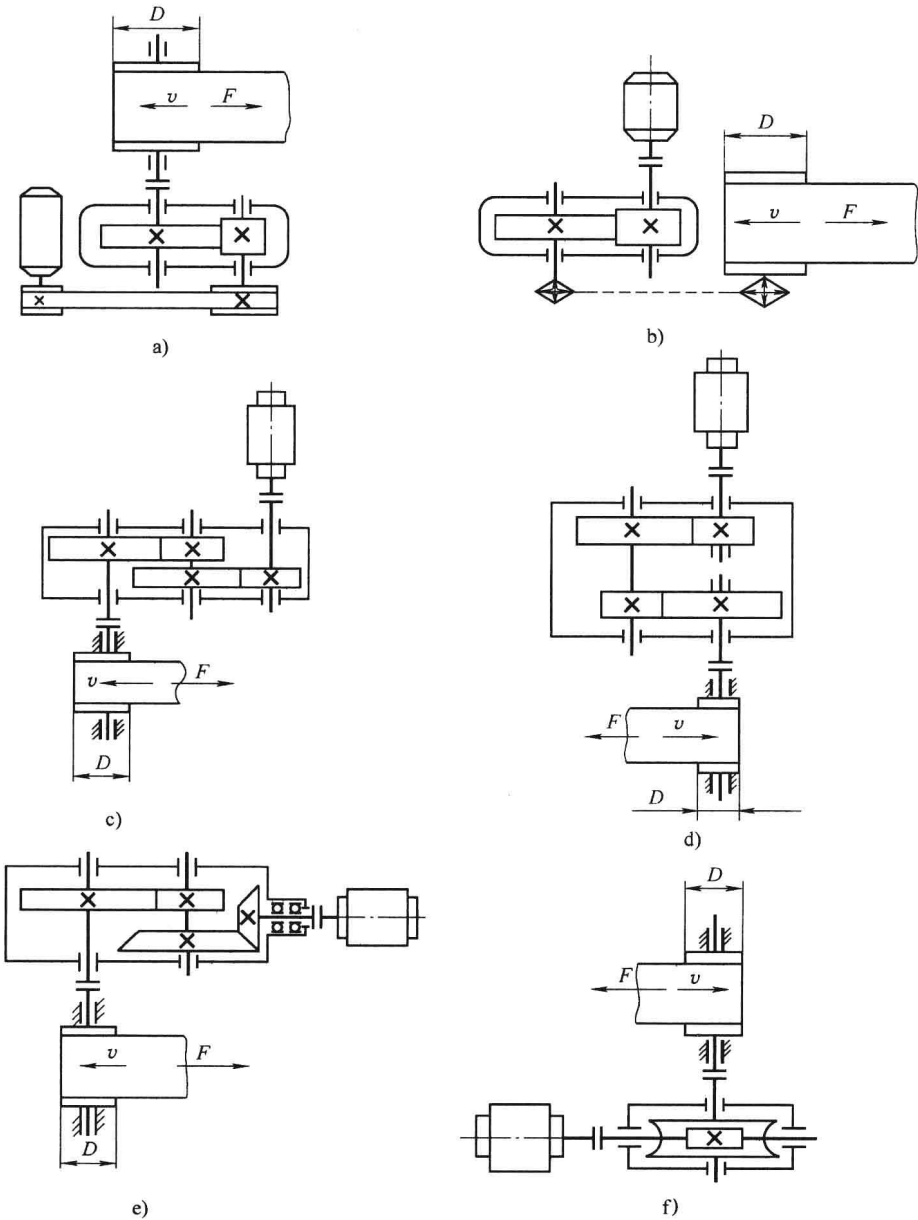
图 1-3 带式输送机传动方案
