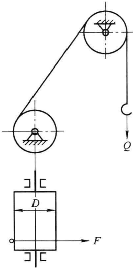
图 1-5 卷扬机工作装置
