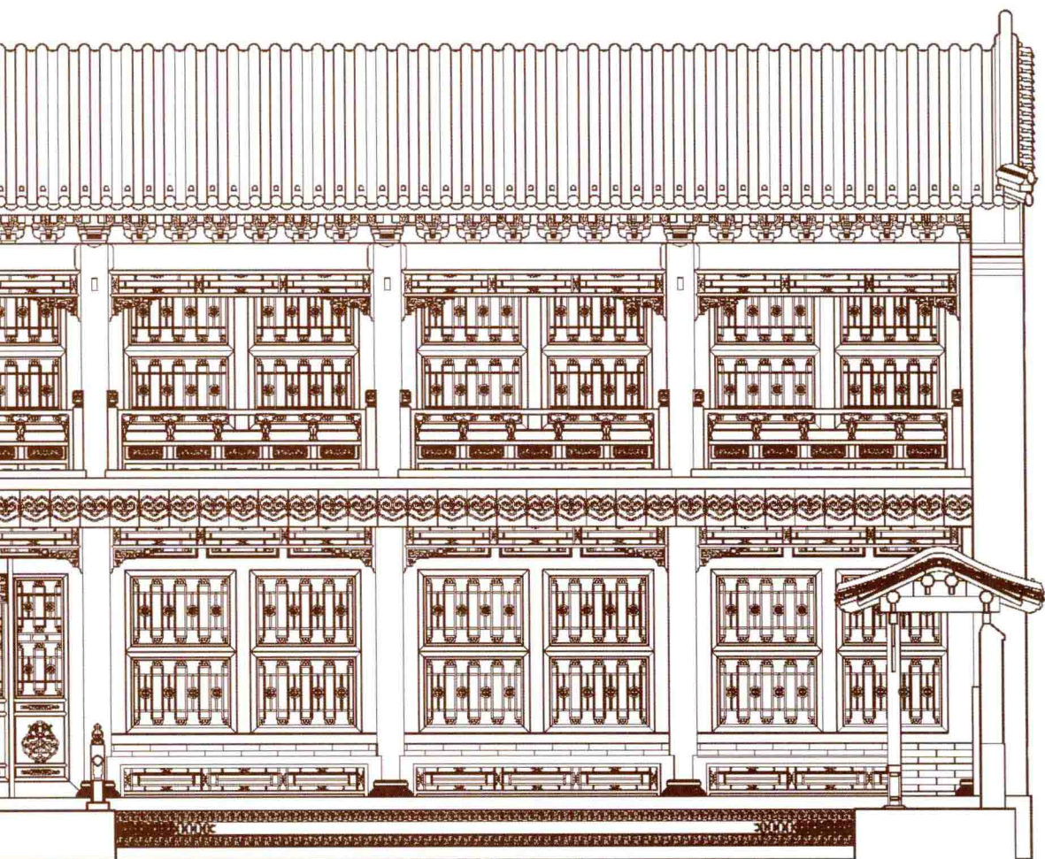
图2 梵华楼正立面图
