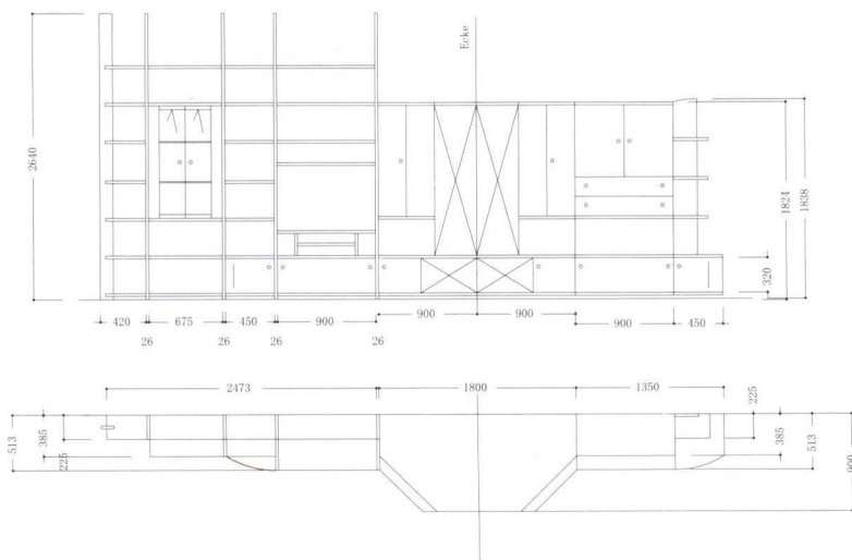
多功能拐角组合声像柜
