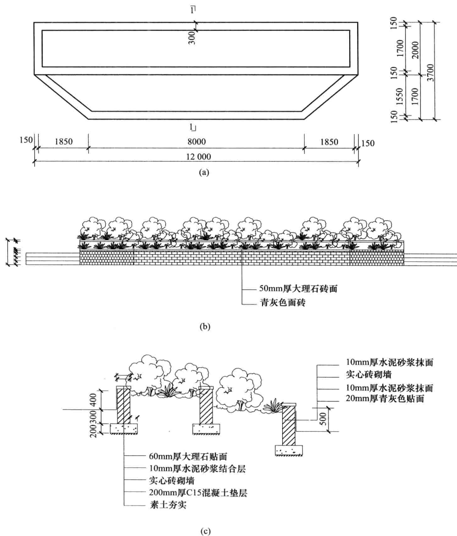
图 1-9 组合花坛
