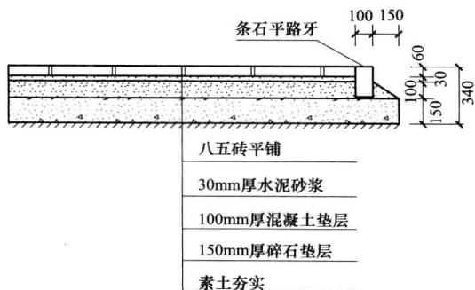
图 1-4 道路剖面示意图 (单位: mm)
