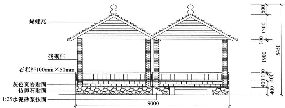
图 1-12(b) 亭子立面图
