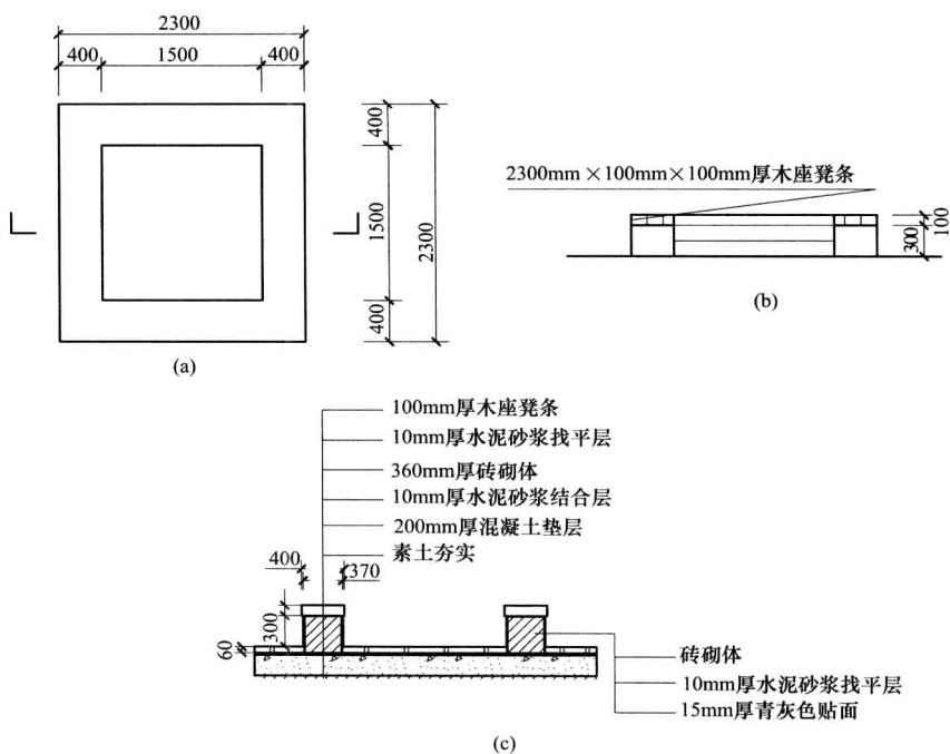
图 1-6 树池
