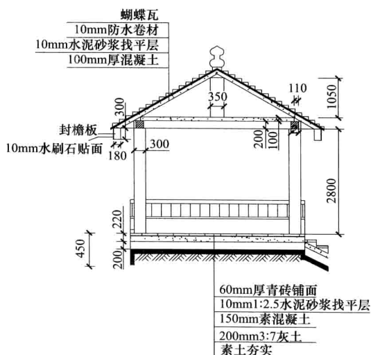
图 1-12(c) 亭子剖面图
