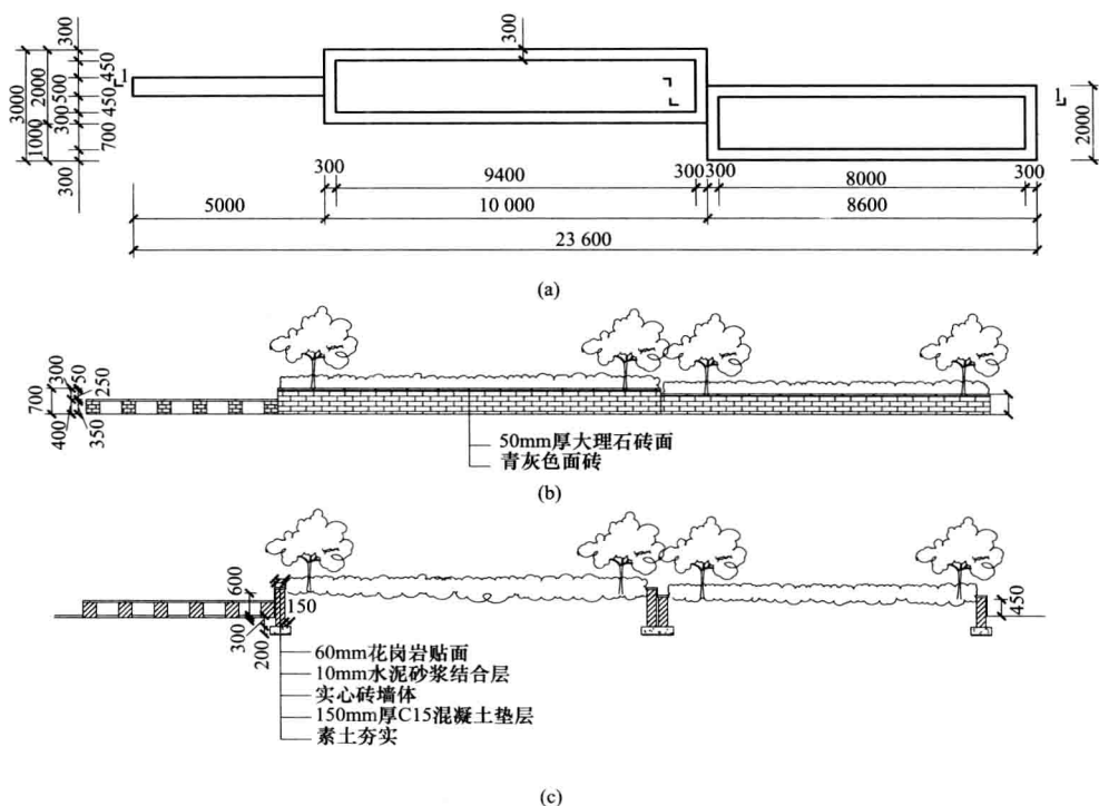
图 1-11 花坛座凳 2
