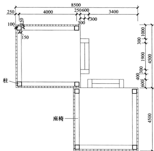
图 1-12(a) 亭子平面图
