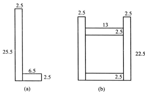
图 1-3 道路平面示意图 (单位: m)
