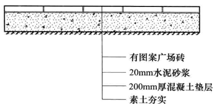
图 1-7 广场剖面图
