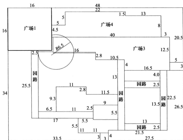
图 1-2 绿地缩略尺寸图 (单位: m)
