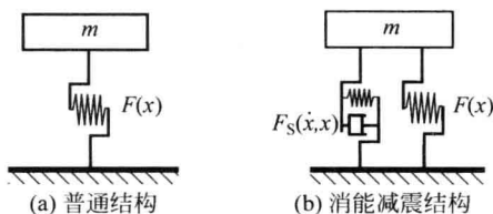
图 2-1 单自由度系统示意图
