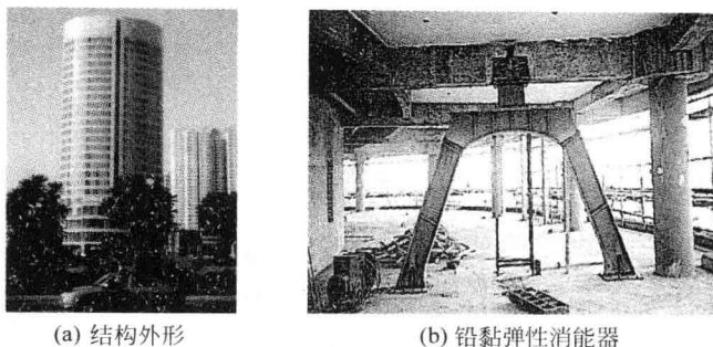
图 1-6 潮汕星河大厦
