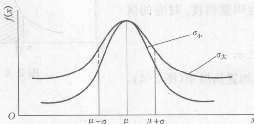
图 2-3 正态分布
