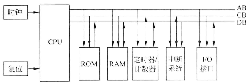
图 1.1 单片机的系统结构
