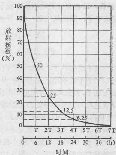
图 1-6 (普通坐标)
