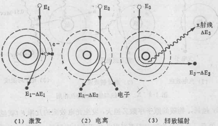
图 1-7 带电粒子与物质的相互作用
