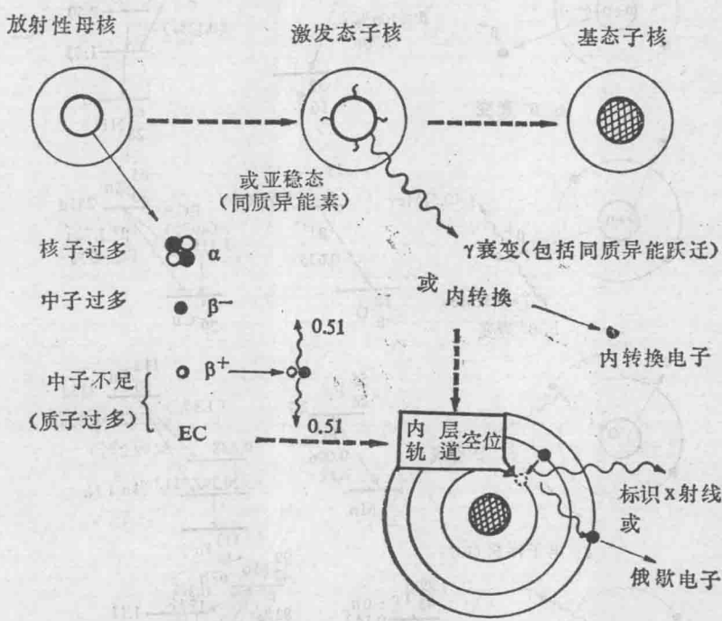
图 1-3 核衰变示意图
