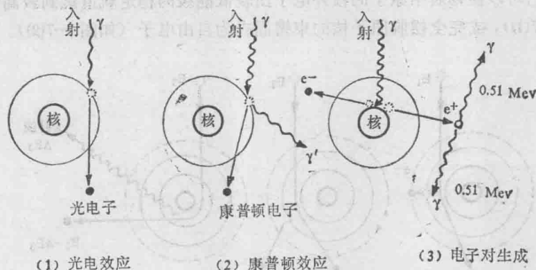
图 1-8 X、 \gamma 射线与物质的相互作用
