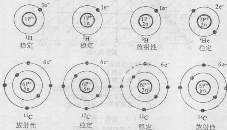
图 1-1 核素示意图
