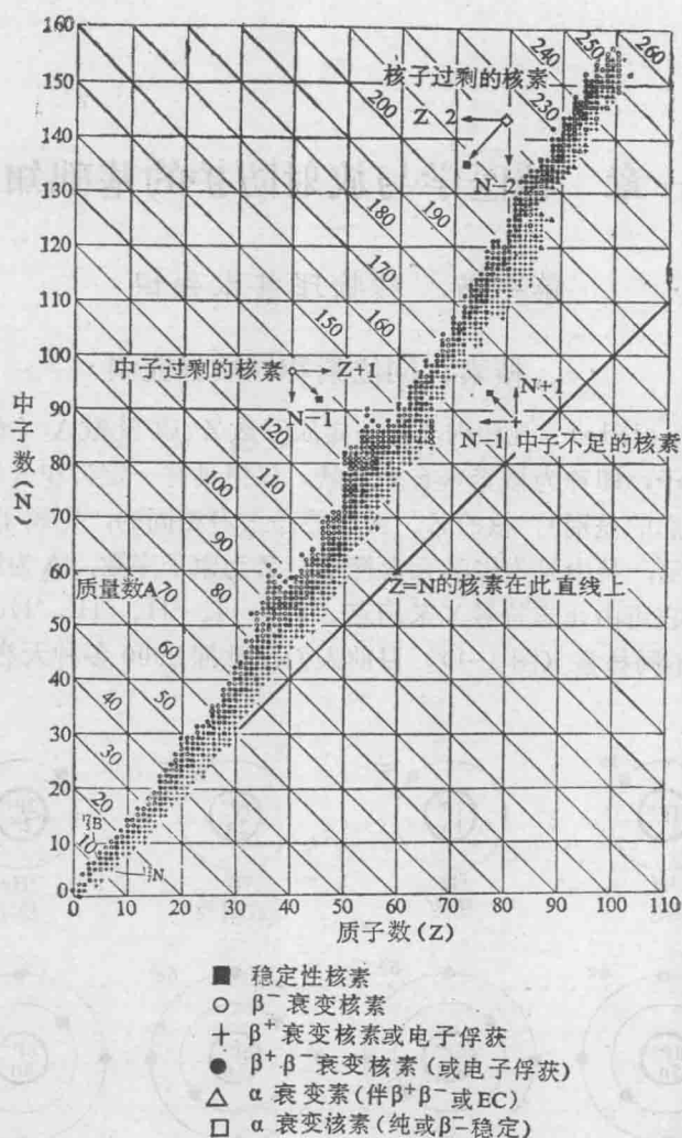
图 1-2 核素一览图 (各种核素的质子和中子组成图)
