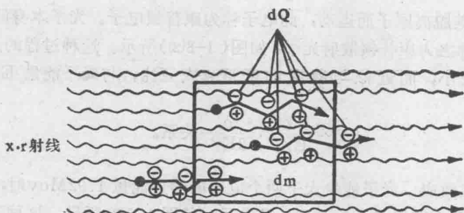
图 1-9 照射量示意图
