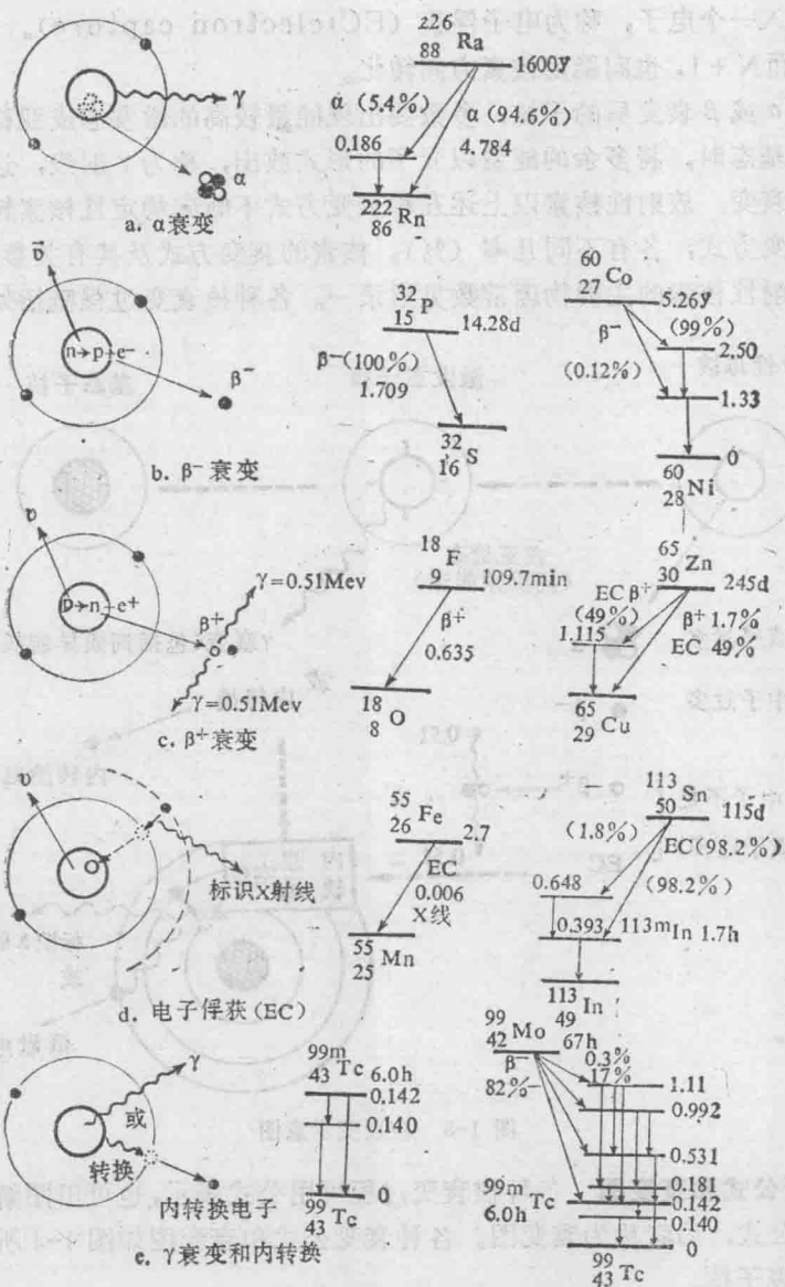
图 1-4 核衰变模式和衰变图
