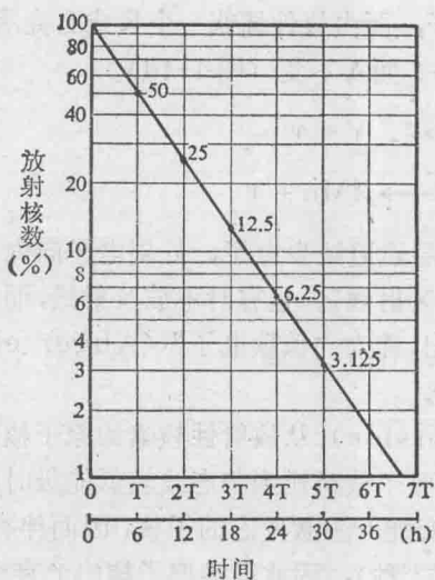
图 1-5 (半对数坐标)
