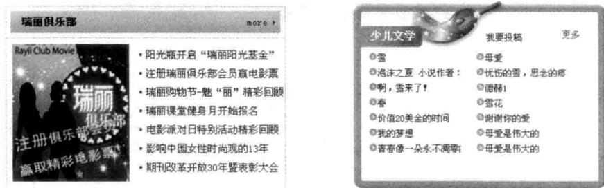
图 1-3 标题栏
