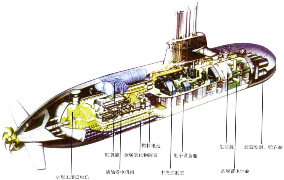
德国 212 型潜艇布置示意图
