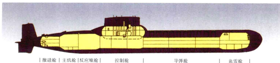
俄罗斯“台风”级核潜艇舱室布置图
