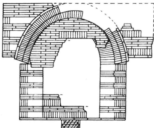
图一四 M12 封门墙剖面图
